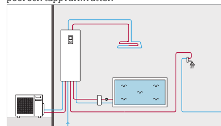
Uppvärmning med golvvärme, uppvärmning av pool och tappvarmvatten
