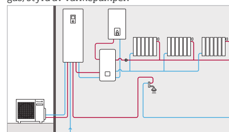
2 värmekällor: Värmepump med oljebrännare eller gas, styrd av värmepumpen
